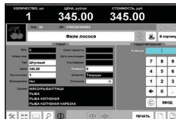
интерфейс оператора
