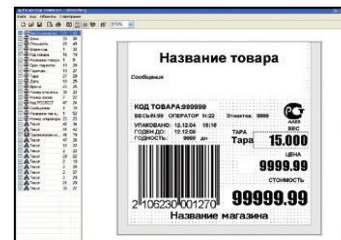
редактор этикеток
